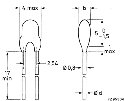
Fig. 1 0,1 W types.
