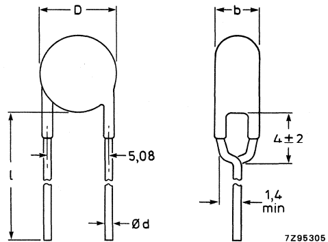
Fig. 2 0,25 and 0,75 W types.
