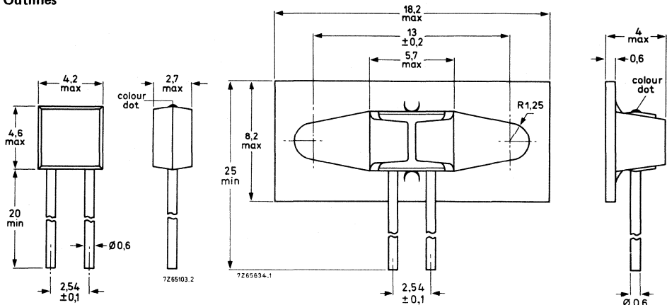
Fig.1 Type 2322 640 90015.
